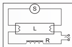
S-starter L-lamp R-ballast
